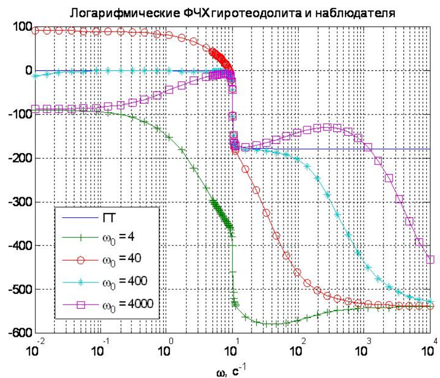
Рис.2. Графики логарифмических частотных характеристик.
