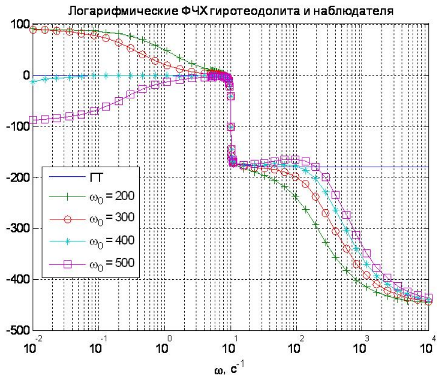
Рис.3. Графики логарифмических частотных характеристик с коррекцией.
