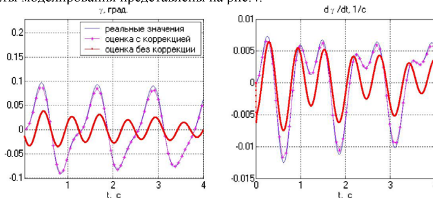
Рис. 4. Моделирование наблюдающего устройства.
