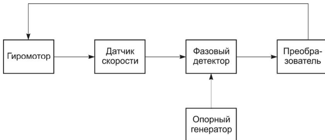
Рис.1. Функциональная схема системы стабилизации.
